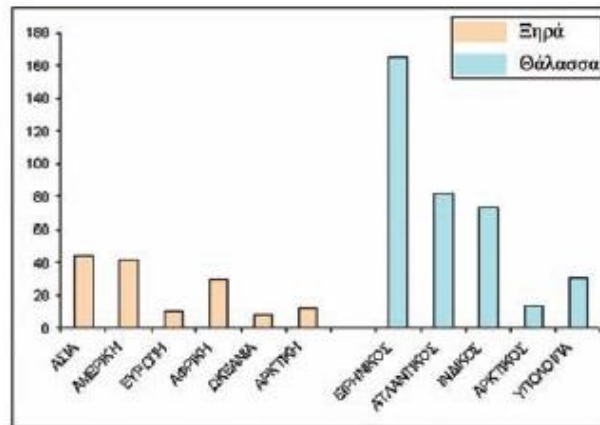
Εικόνα 7.3α: Κατανομή Ξηράς και θάλασσας
