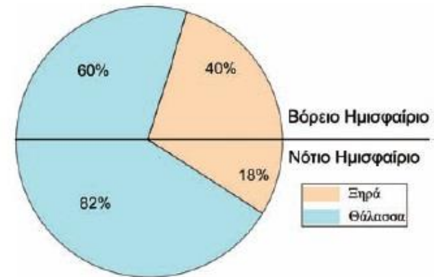
Εικόνα 7.3β: Κατανομή Ξηράς και θάλασσας στα ημισφαίρια
